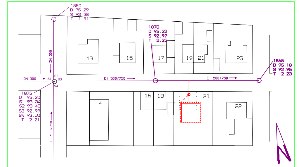
Lageplan M 1:1000
